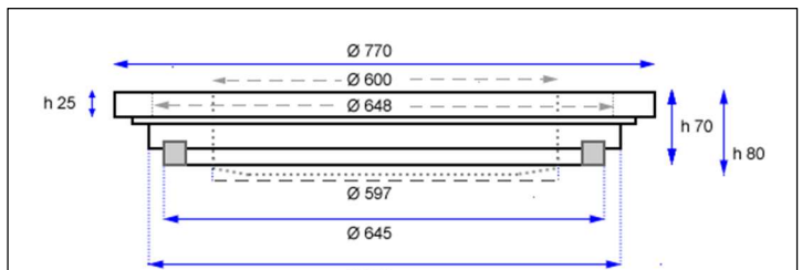
Skizze Swiss-Edition DN 600 35kN mit CH-Modulrahmen – Abmessungen ca. Angaben
