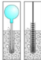
2. Bohrloch reinigen mit Sauger oder Bürste
