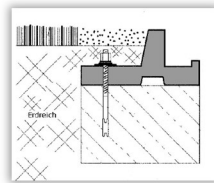
DN 600 BASIC Flanschrhahmen für flache Montage auf Schacht mit LW 60 cm
